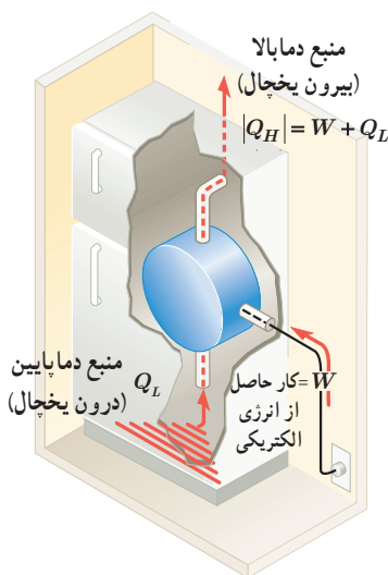
شکل ۵-۲۱ طرحی از طرز کار یک یخچال خانگی
