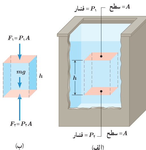
شکل ۲-۱۴ الف) بخشی از شماره ساکن (ب) نیروهای وارد بر این بخش از شماره در راستای قائم.
